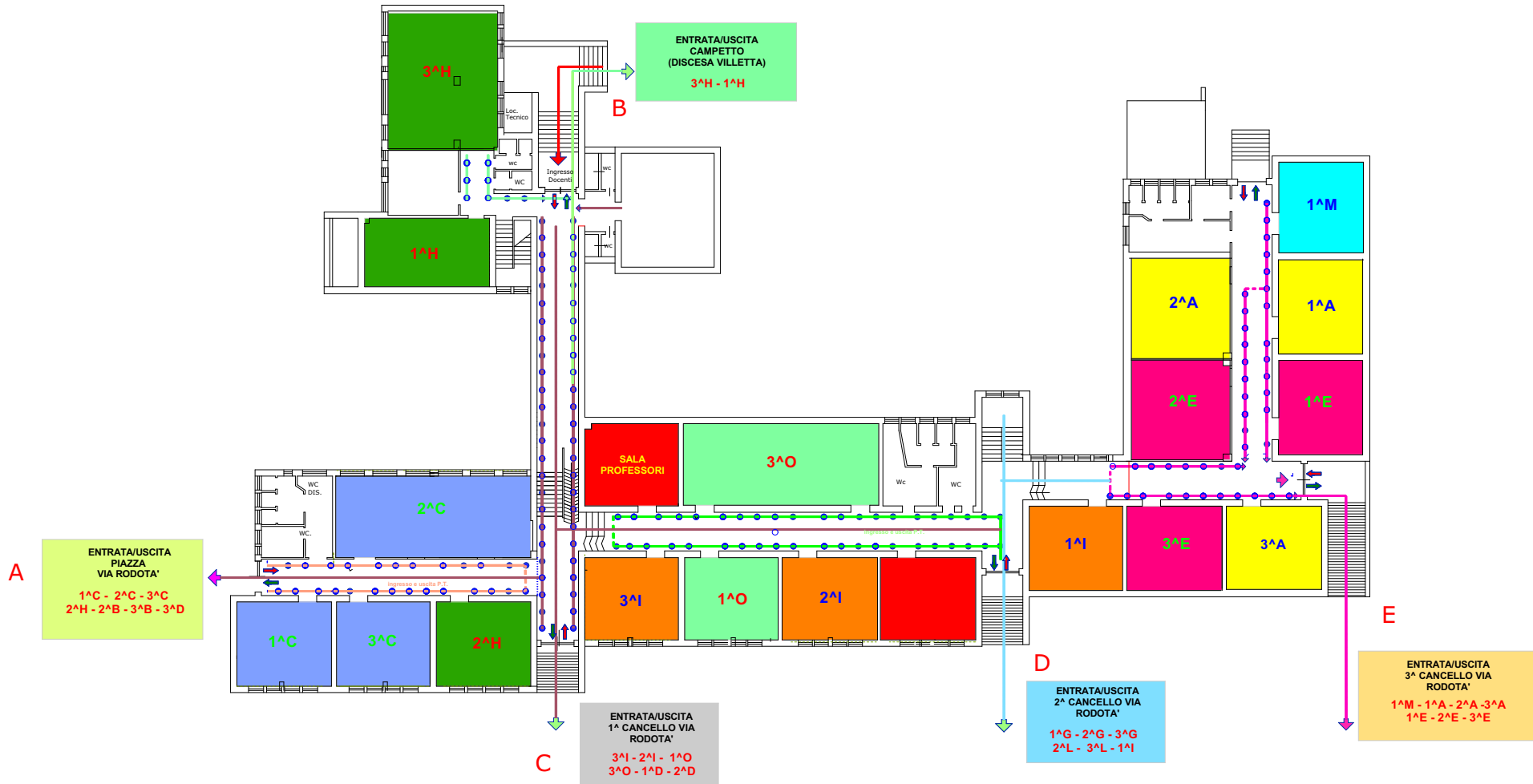
PIANTA PIANO TERRA INGRESSI/USCITE
